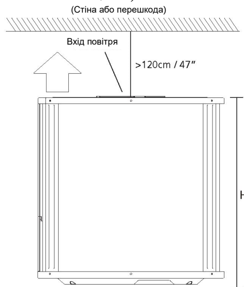
Зовнішній блок з вертикальним нагнітанням (див. Мал. 5.7 5.8 5.9 і таблицю 5.2)
