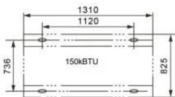
Отвори для кріплення 15*20мм
