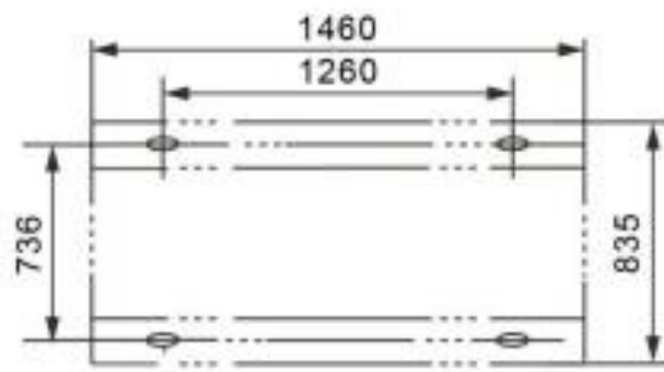
Отвори для кріплення 15*20мм
